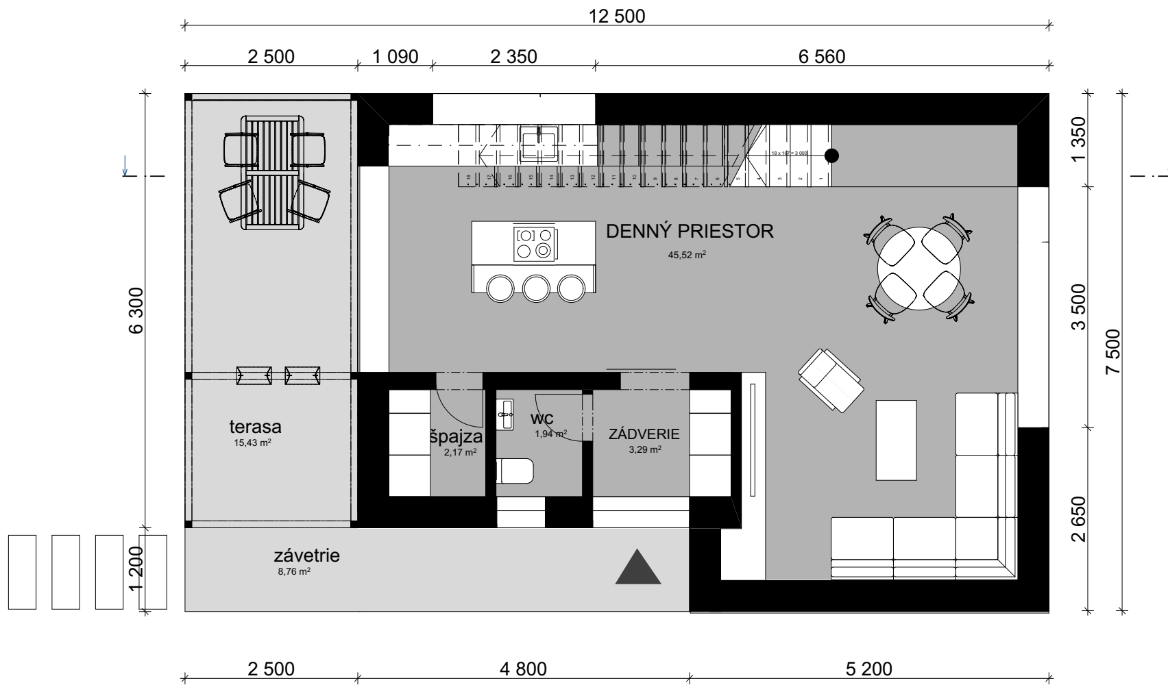
pôdorys 1np
